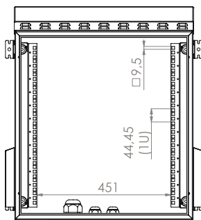
Innenansicht
