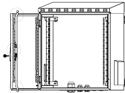
3-Punkt-Verriegelungssystem
