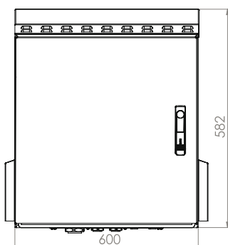
Frontansicht
