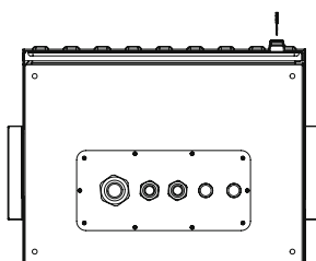
Bodenansicht
